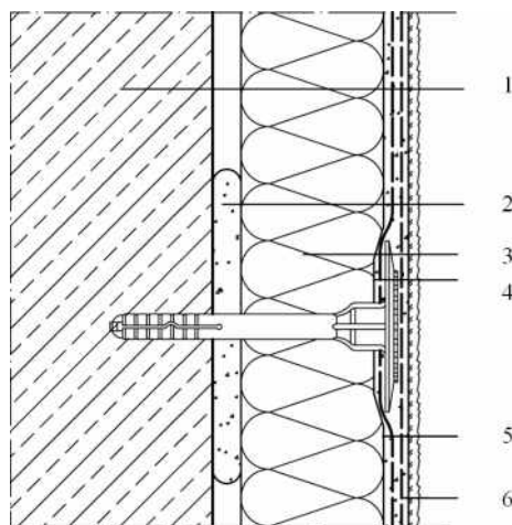
图 5.4.5-2 岩棉板双网构造示意图
