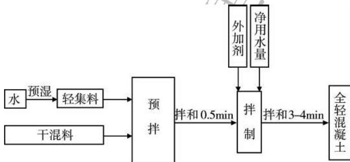
图 5.3.4-1 使用预湿处理轻集料时的投料顺序示意图
