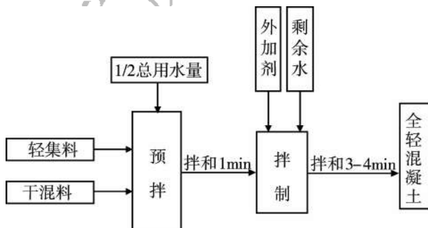
图 5.3.4-2 使用未预湿处理轻集料时的投料顺序示意图
