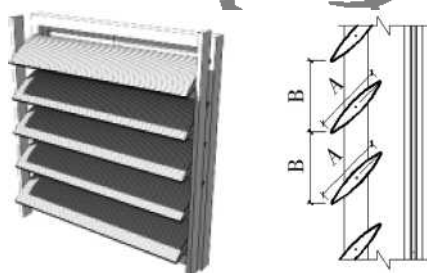
图 C.0.4 横百叶挡板式外遮阳的特征值
