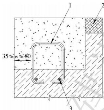
图 5.0.7-1 锚固布置图(一)(单位:mm)
