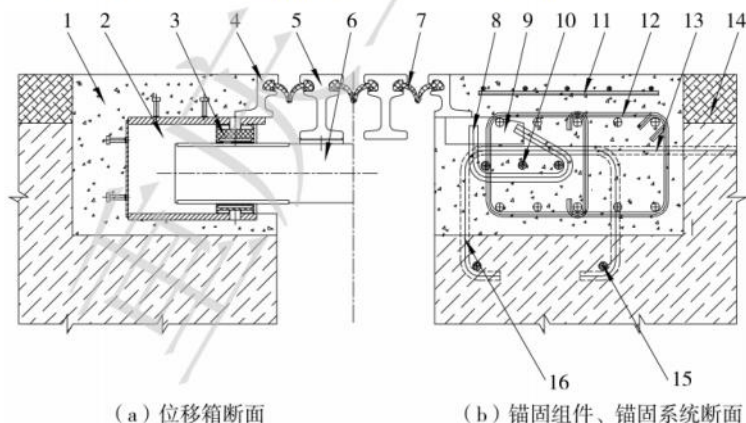
图 4.0.2 多缝伸缩装置锚固构造截面示意图
